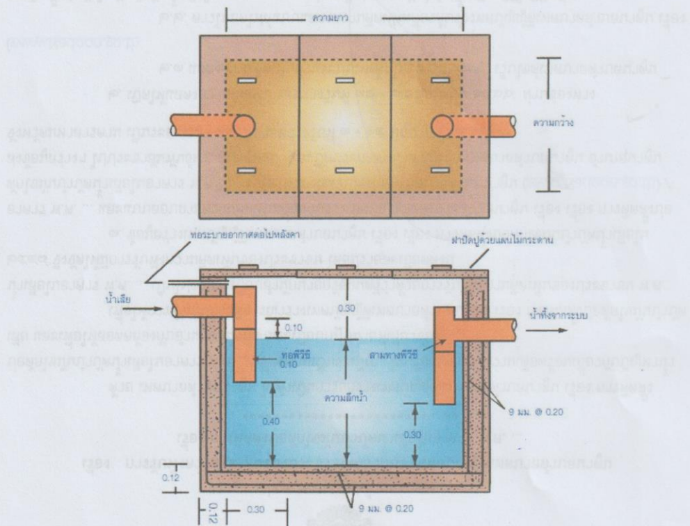
บ่อดักไขมันแบบสร้างในที่สำหรับอาคารขนาดใหญ่
